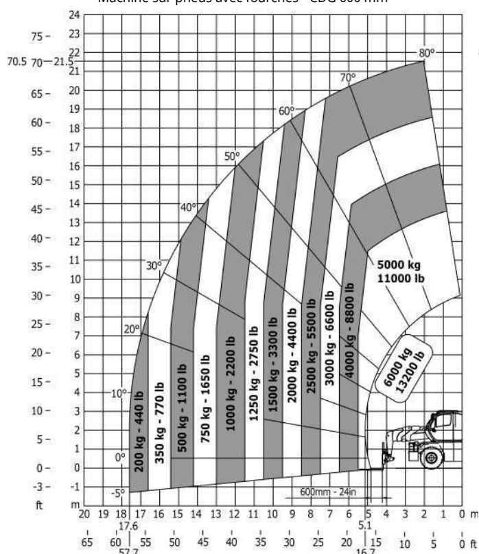
Machine sur pneus avec fourches - CDG 600 mm
