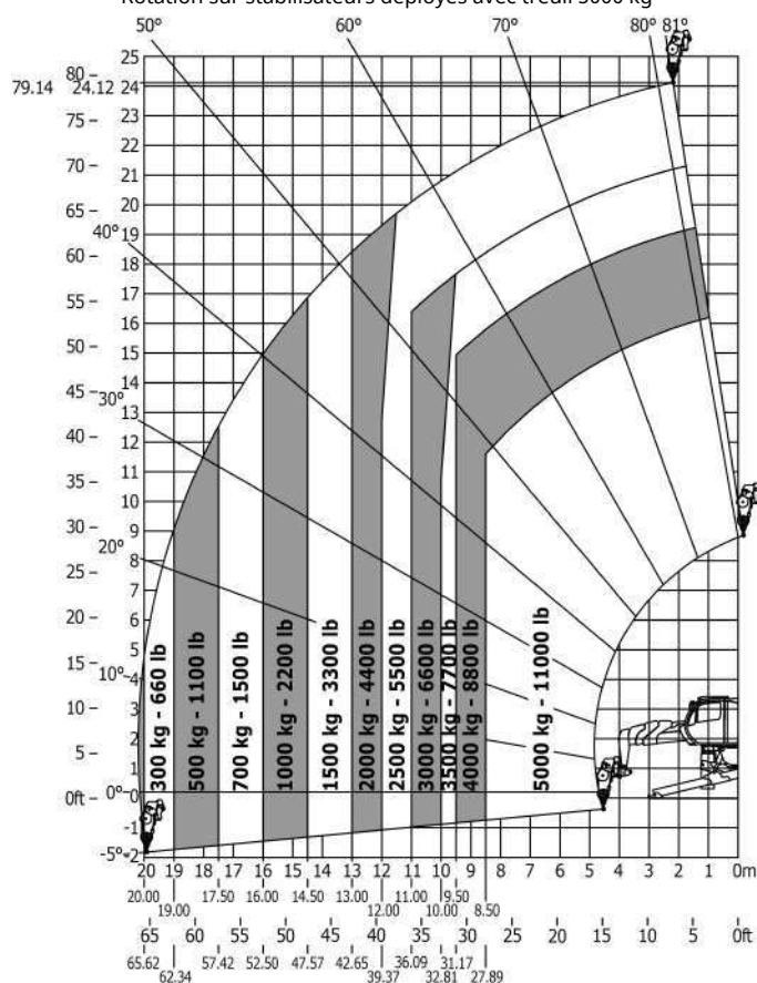
Rotation sur stabilisateurs déployés avec treuil 5000 kg
