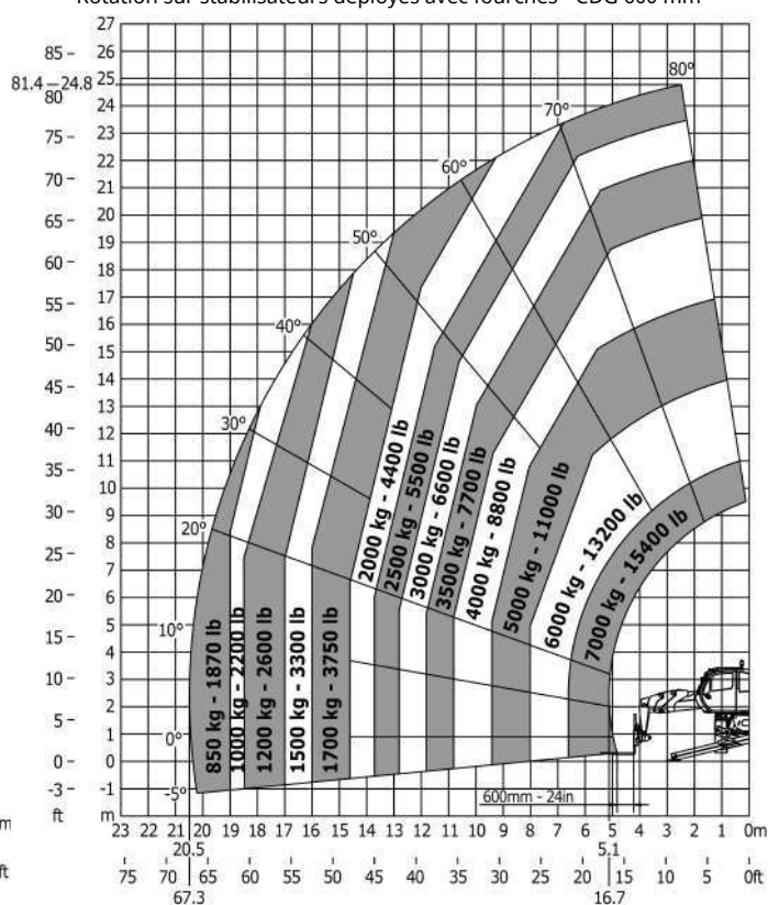
Rotation sur stabilisateurs déployés avec fourches - CDG 600 mm
