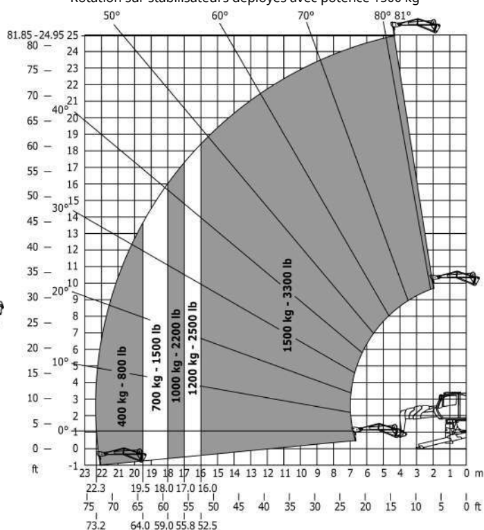
Rotation sur stabilisateurs déployés avec potence 1500 kg
