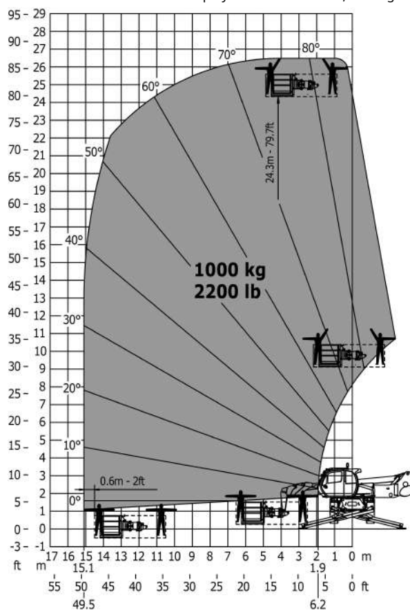
Rotation sur stabilisateurs déployés avec nacelle 365/1000 kg
