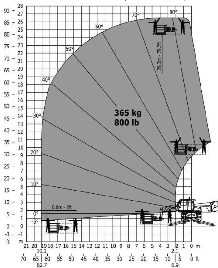
Rotation sur stabilisateurs déployés avec nacelle 365 kg
